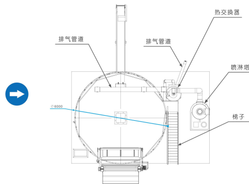
1 发酵罐顶视图 Top view
