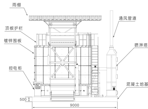
2 发酵罐正视图 Front view
